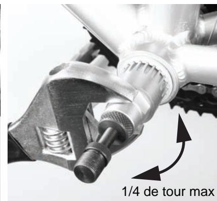
4 Faites tourner la douille au maximum d'un quart de tour à l'aide de la clé pour desserrer la cuvette de pédalier, puis enlevez le BBSH-1 du jeu de pédalier.
