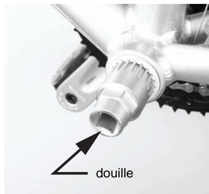
2 Installez la douille comme illustré.
