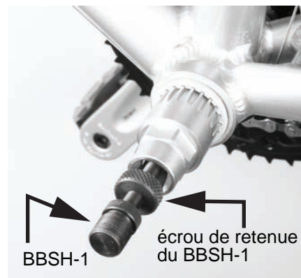
3 Installez le BBSH-1 et l'écrou de retenue de douille comme illustré. Assurez-vous que l'écrou de retenue et la douille sont bien ajustés.
