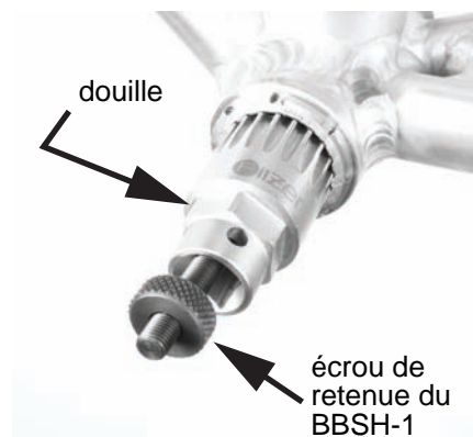
3 Installez la douille et son écrou de retenue comme illustré. Assurez-vous que l'écrou de retenue et la douille sont bien ajustés.
