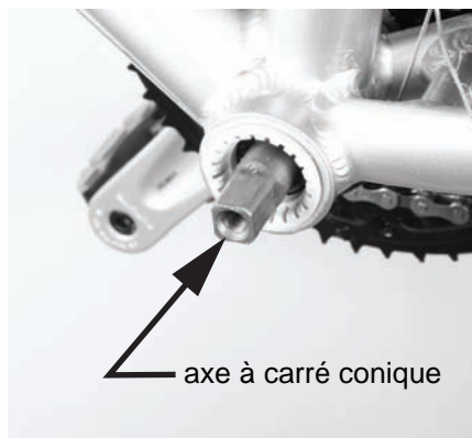
1 Retirez la manivelle.
