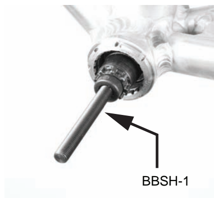
2 Installez le BBSH-1 comme illustré.
